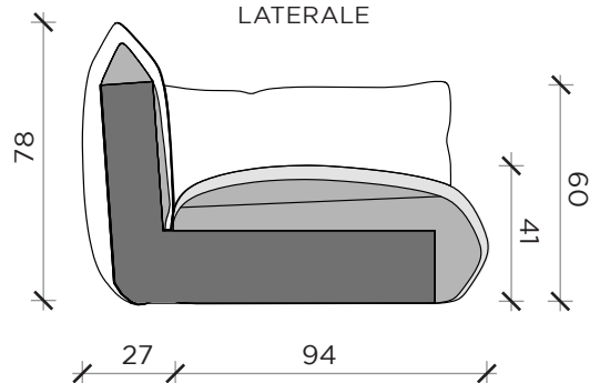
SEZIONE LATERALE
